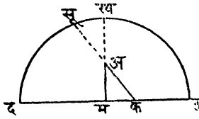
अक्षक्षेत्र व पलभा दाखविणारी आकृति.
